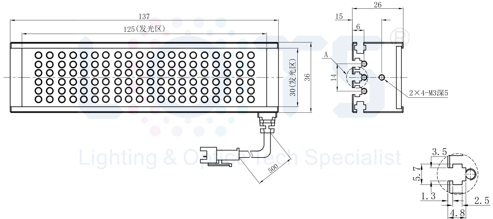
视图A
